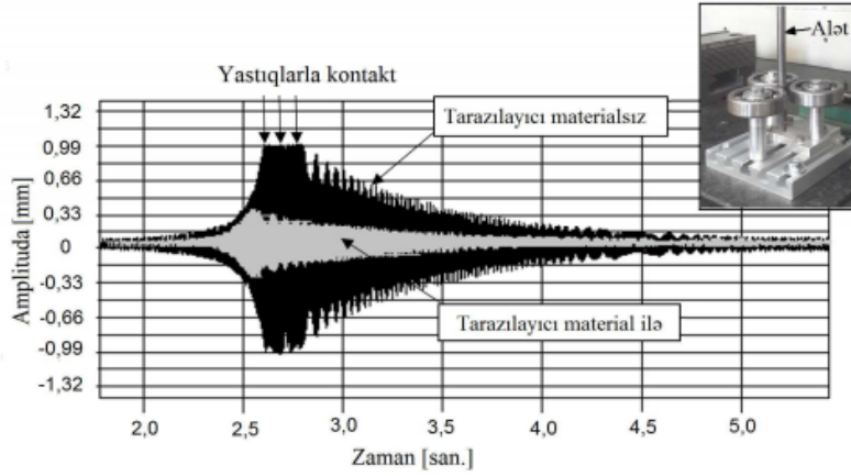
Şəkil 2. Tarazlayıcı materialın frez alətinin yırğalanmasına təsiri [1]
